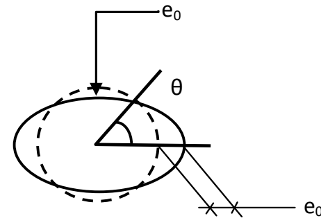
Figure 10 : Définition du défaut initial de forme
